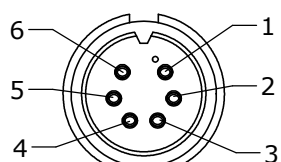
FACE VIEW P/N: 3282-6SG-5XX
