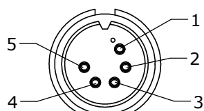
FACE VIEW P/N: 3282-5SG-5XX
