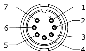
FACE VIEW P/N: 3282-7SG-5XX
