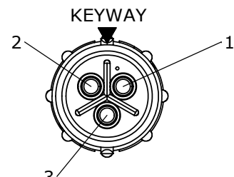
WIRE VIEW 8380-3SG-3XX
