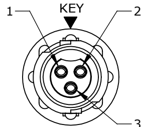
FACE VIEW W18282-3SG-P-5XX
