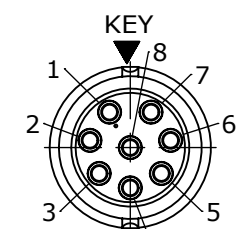
WIRING END W6280-8SG-P-3XX
