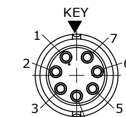
WIRING END W6280-7SG-P-3XX
