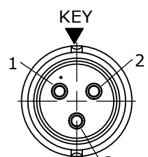
WIRING END W6280-3SG-P-3XX
