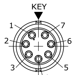
WIRING END W6282-7SG-P-5XX
