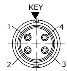
WIRING END W6282-4SG-P-5XX
