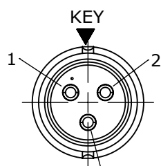
WIRING END W6282-3SG-P-5XX
