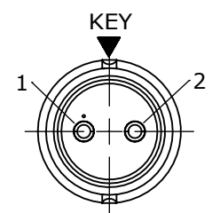
WIRING END W6282-2SG-P-5XX
