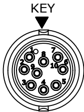
WIRING END W6880-9SG-P-5XX
