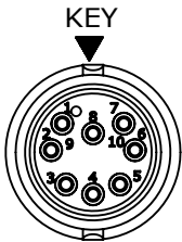
WIRING END W6880-8SG-P-5XX
