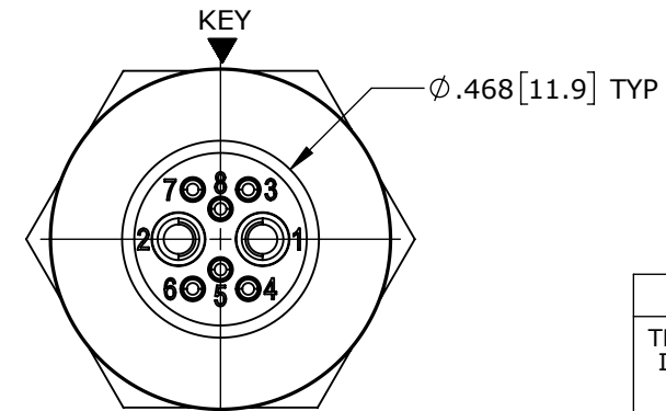
WIRING END W7A82-8PG-P-300 SHOWN
